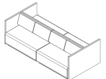
MODULE 6 2600(L) X 1300(D) X 850(H)
