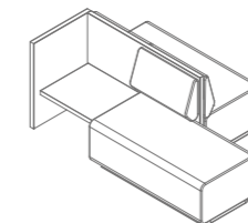
MODULE 5 1950(L) X 1300(D) X 850(H)
