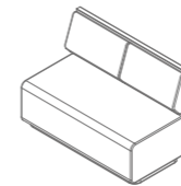
MODULE 1 1300(L) X 650(D) X 850(H)
